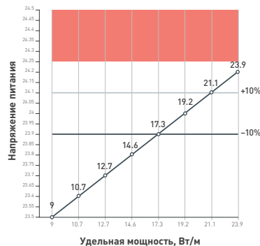
График 1. Зависимость удельной мощности от напряжения питания
