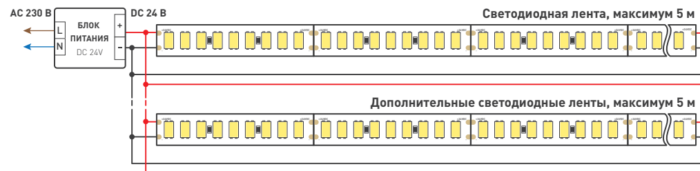
Схема 2. Подключение нескольких светодиодных лент с двух сторон для обеспечения равномерного свечения ленты по всей длине
