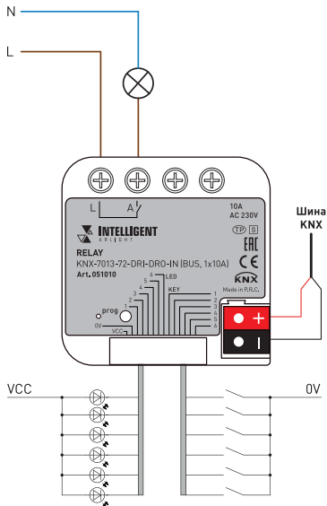
Рис. 1. Пример схемы подключения оборудования
