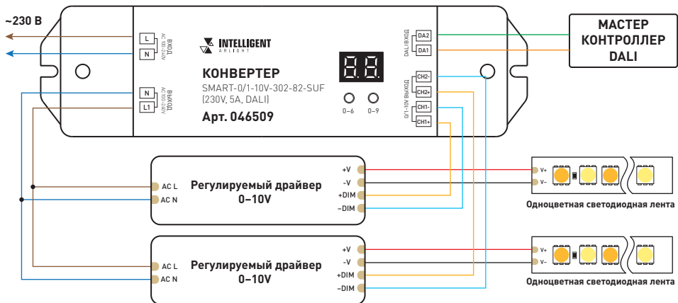
Рис. 2. Схема подключения конвертера при использовании выхода реле
