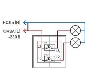
Рис. 1. Схема подключения (арт. 043724, 043725, 043726)
