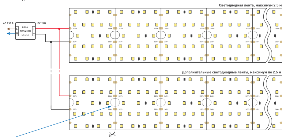
Схема 1. Подключение нескольких светодиодных лент
