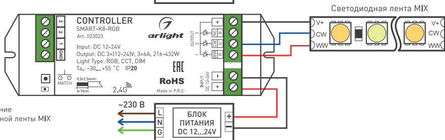
Рисунок 1. Подключение светодиодной ленты RGB
