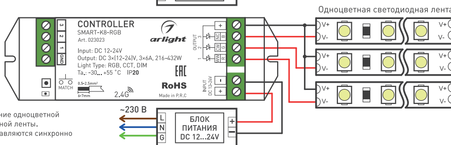
Рисунок 2. Подключение светодиодной ленты MIX
