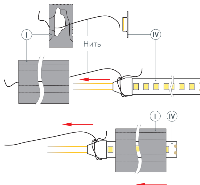
Рис. 1. Протяжка светодиодной ленты ④ в профиль ①, вид сбоку
