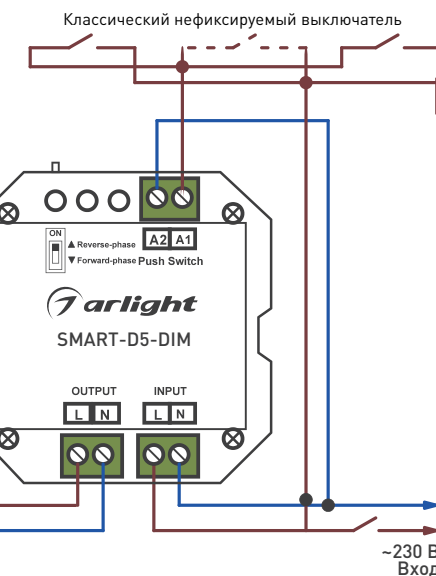
Рисунок 1. Типовая схема подключения диммера
